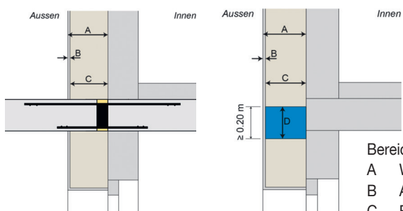
Detail mit BASYCON Anschluss RF1
