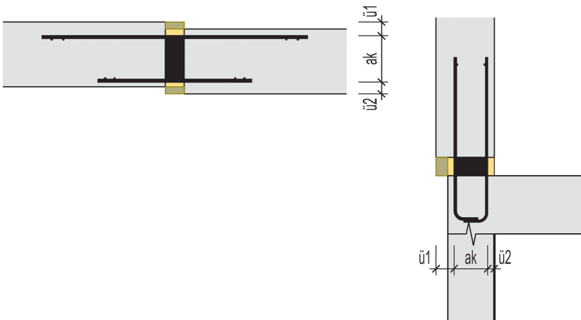
Aufdoppelung Isolation
