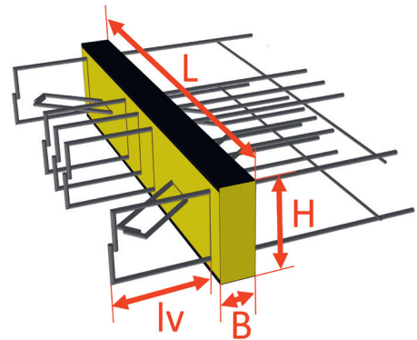
Brüstungsanschlüsse
