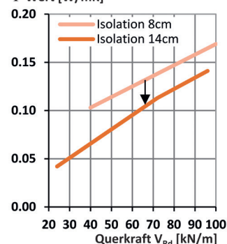
Beispiel Querkraftanschlüsse Wärmebrückenzuschlag \Psi -Wert [W/mK]
