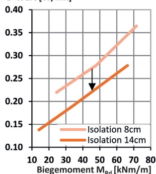
Beispiel Kragplattenanschlüsse Wärmebrückenzuschlag \Psi -Wert [W/mK]
